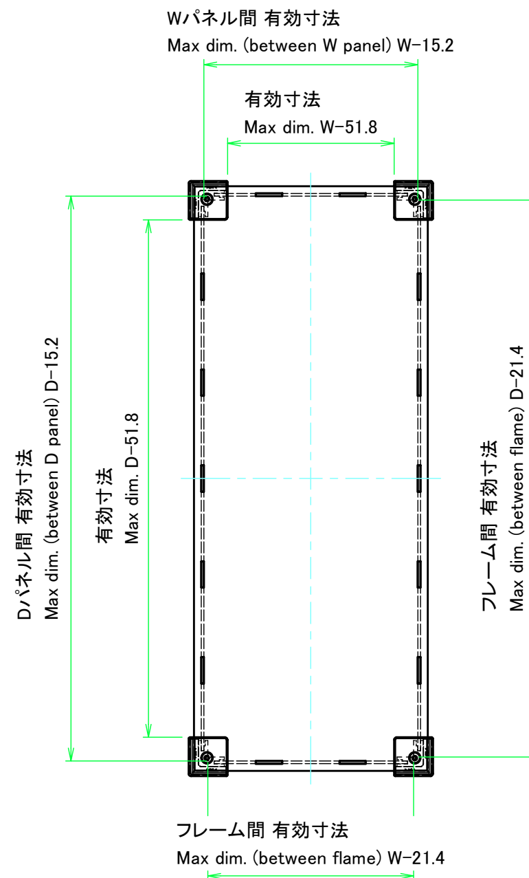
下カバー / Bottom cover
