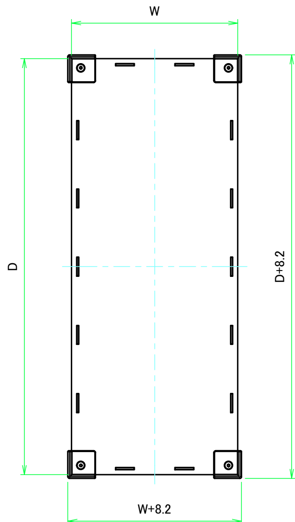
Wパネル1 / W Panel 1
