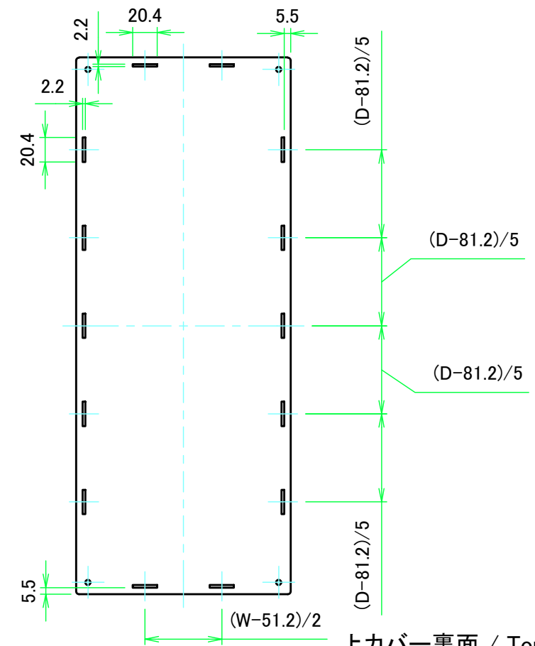
上カバー裏面 / Top cover Backside
